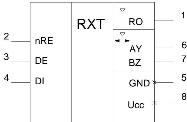
Рисунок 2 – Условное графическое обозначение
