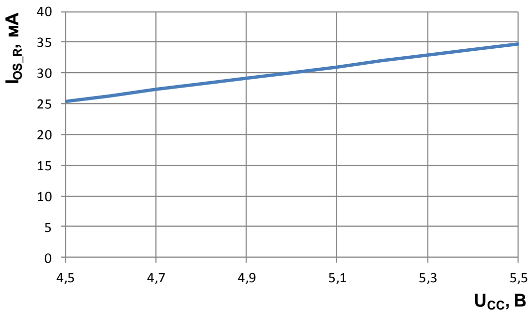
Рисунок 5 – Зависимость тока короткого замыкания выхода приемника I_{OS\_R} от напряжения источника питания при T = 25 °С
