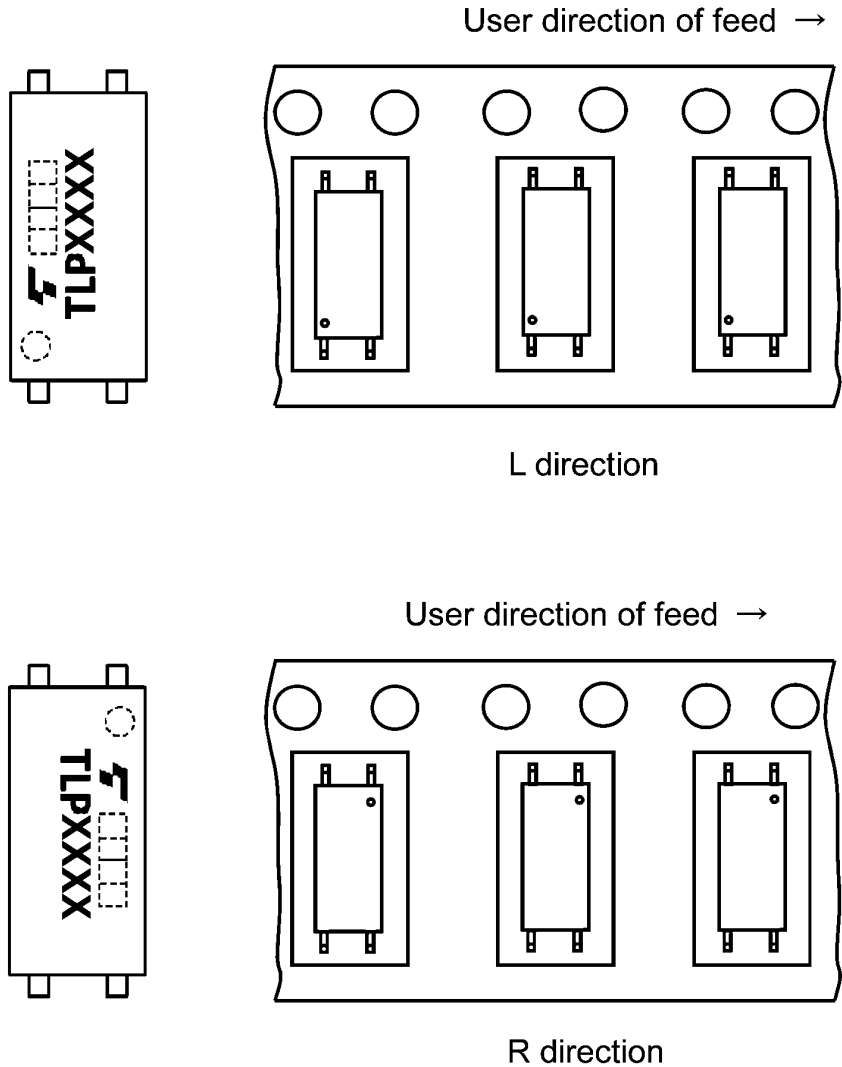
Fig. 16.3.1.1 Device Orientation
