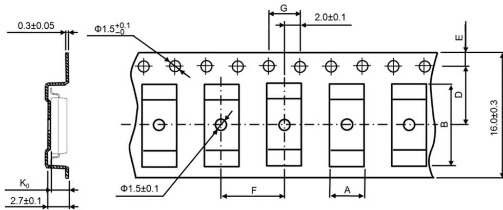
Fig. 16.3.5.1 Tape Dimensions
