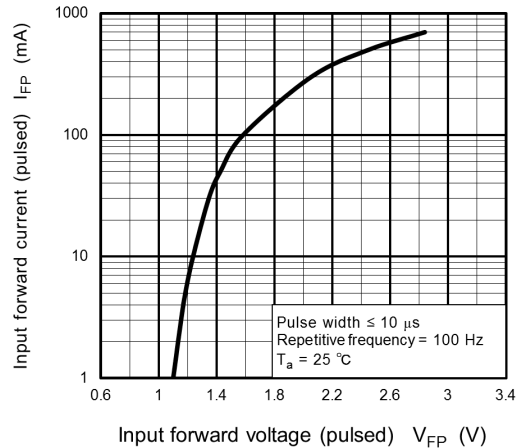
Fig. 11.6 I_{FP} - V_{FFP}
