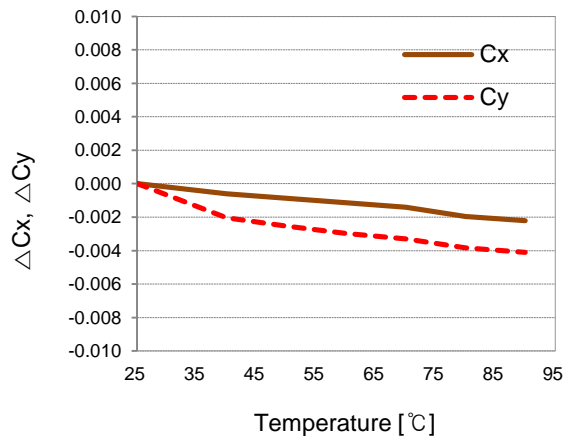
■ CIE vs. Temp.
