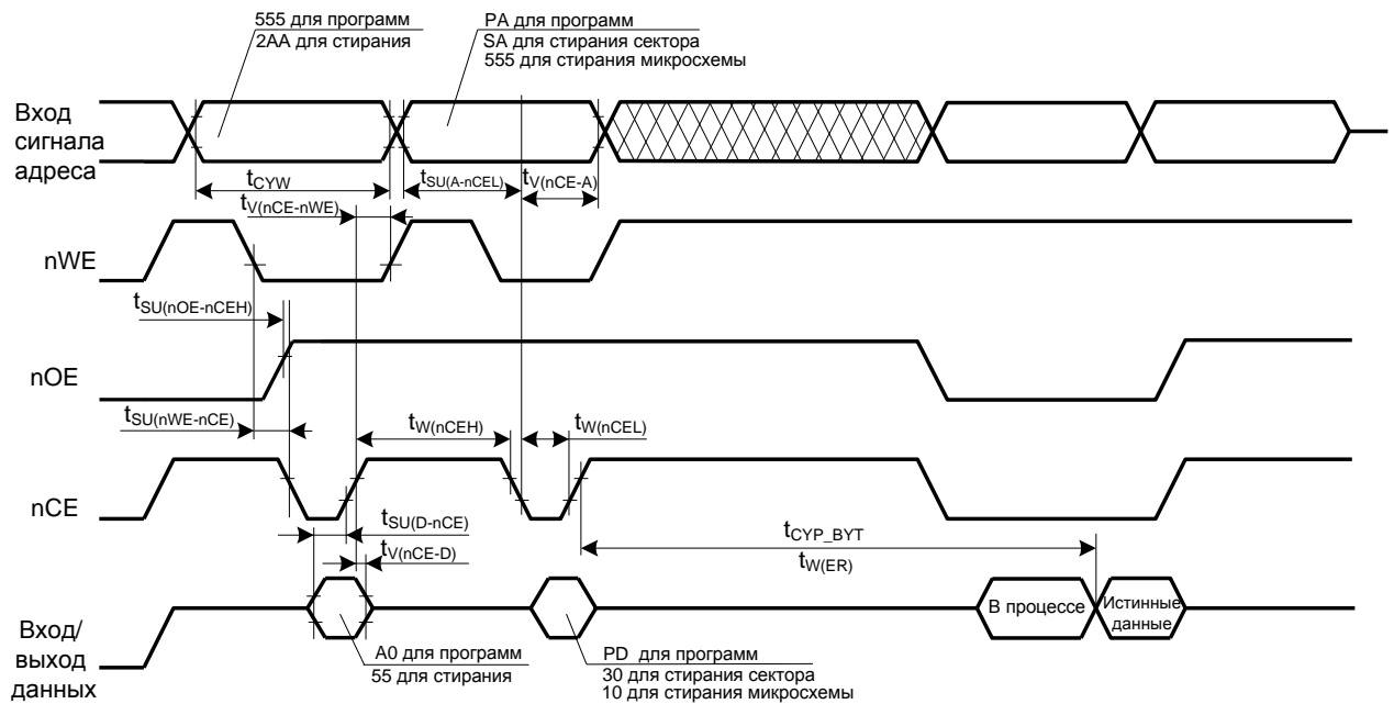
Рис.13 Временная диаграмма цикла записи 1. Управление по nWE. U_{nOE}=U_{IH} на протяжении цикла записи
