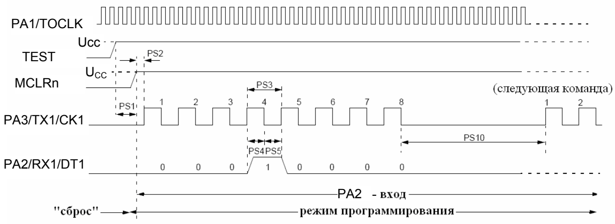
Рисунок 7 – Команда программирования
