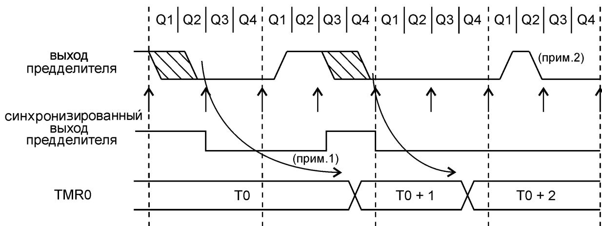
Рис. 25 Функционирование «таймер 0» от внешнего источника тактовых импульсов
