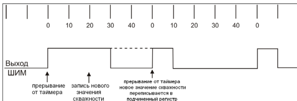
Рис. 30 Выход ШИМ
