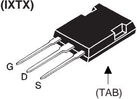
PLUS247 (IXTX)
